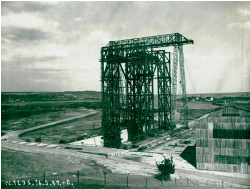
Metallskelett des alten Schiffshebewerks
