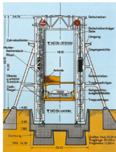
Querschnitt des alten Schiffshebwerks
