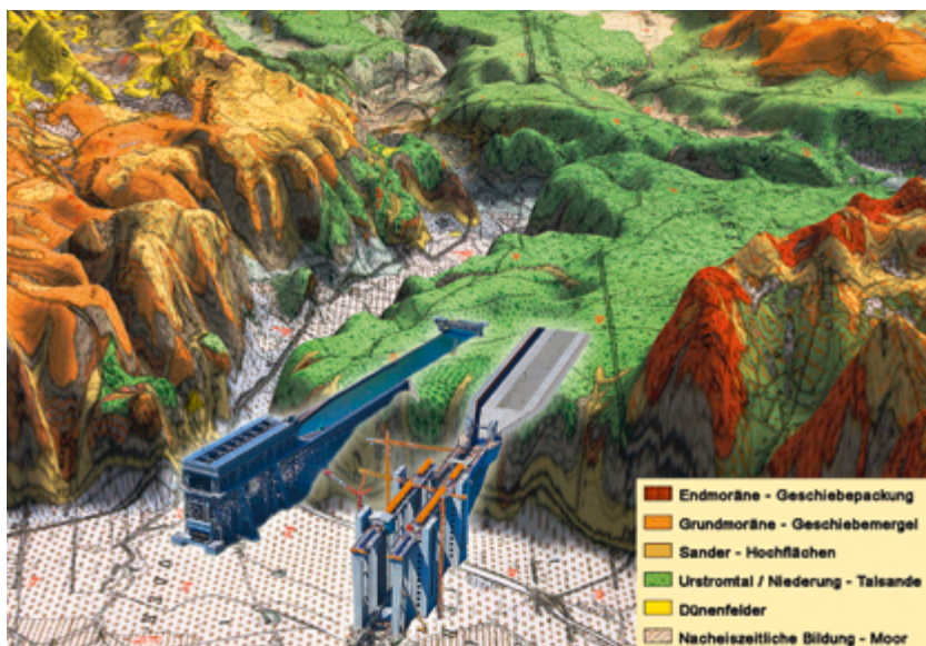
Die Hebewerke gleichen den Geländesprung zwischen Urstromtal und der Platte des Barnims aus (Illustration: Dr. Gerd Lutze/Märkische Eiszeitstraße e.V.)
